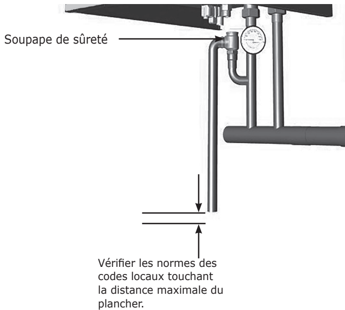
FIGURE 5-2 Canalisation de sortie de la soupape de sûreté
