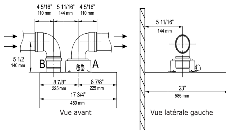
FIGURE 6-9 Options d'installation d'extrémités d'évent horizontales séparées
