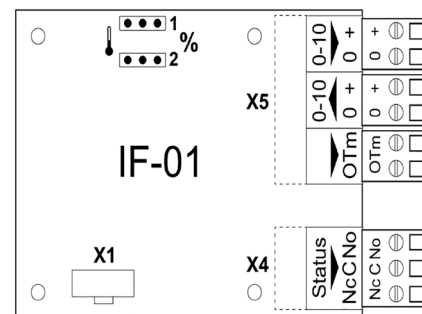
FIGURE 8-6 Commande à carte de circuits imprimés 0 à 10 V (IF-01)
