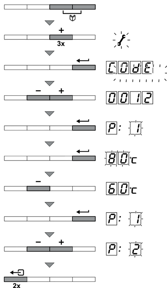
FIGURE 9-10 Paramètres configurables par l'installateur
