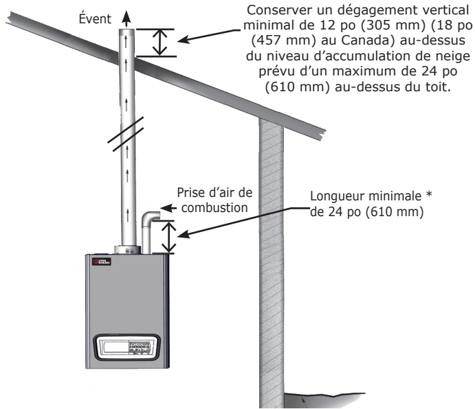
FIGURE 6-20 Évacuation sur le toit, prise d'air nécessaire à la combustion
