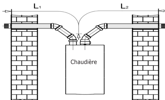
FIGURE 6-9 Options d'installation d'extrémités d'évent horizontales séparées
