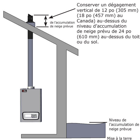
FIGURE 6-3 Événement concentrique pour installation sur le toit
