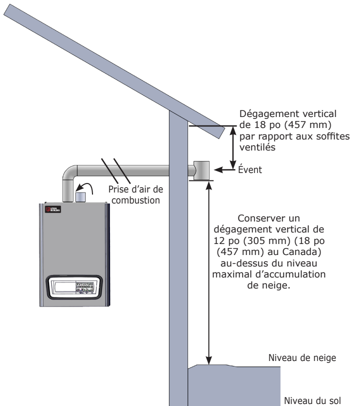
FIGURE 6-21 Évacuation murale, prise intérieure d'air nécessaire à la combustion
