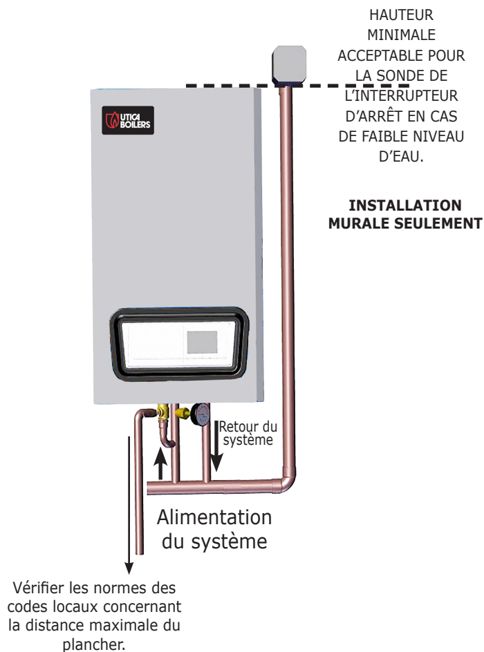
FIGURE 5-3 Canalisations du système : emplacement de la sonde de l'interrupteur en cas de faible niveau d'eau
