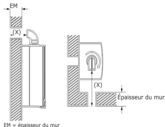
FIGURE 6-2 Événement concentrique pour mur latéral
