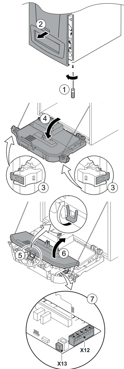
FIGURE 8-2 Retrait du panneau avant
