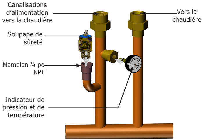
FIGURE 5-1 Soupape de sûreté
