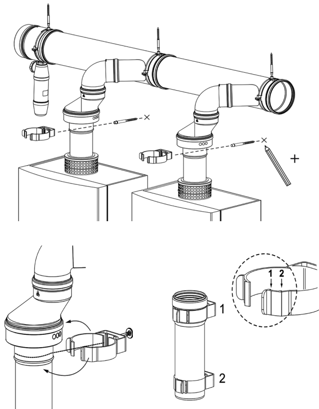
FIGURE 6-32 Fixer la bride autour de l'adaptateur d'évacuation
