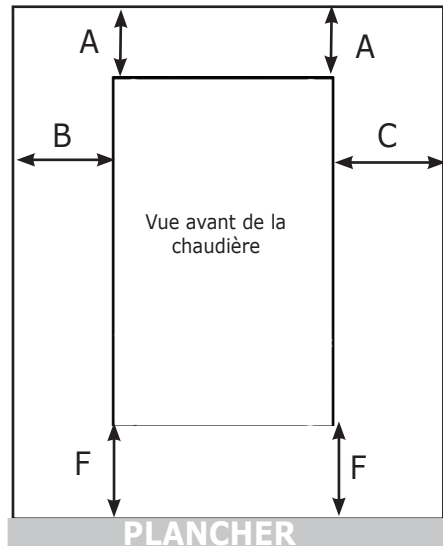
FIGURE 4-1b Dégagement par rapport aux matériaux combustibles
