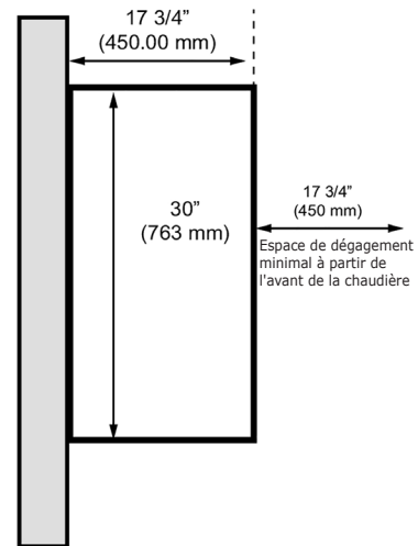
FIGURE 4-2c Dégagement pour l'entretien, installation dans un placard
