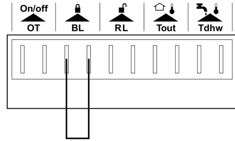
FIGURE 8-4 Signal de dégagement
