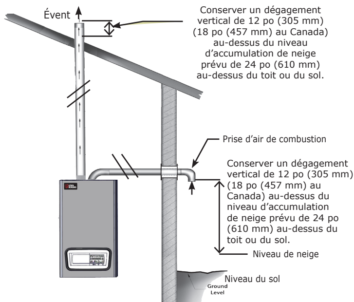
Figure 6-18 Évacuation sur le toit, prise d'air nécessaire à la combustion sur le mur latéral
