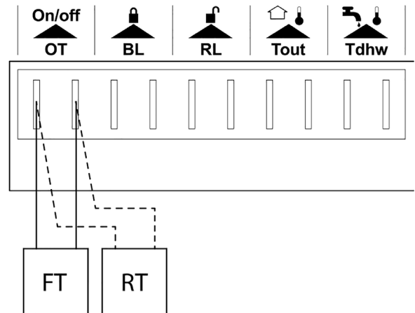
FIGURE 8-13 Protection contre le gel combinée au thermostat de marche/arrêt.
