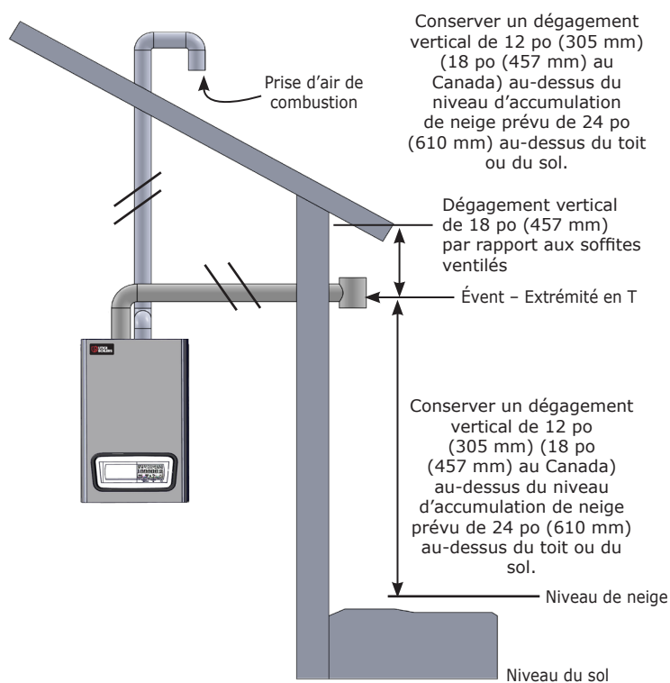
Figure 6-19 Évacuation murale, prise d'air nécessaire à la combustion sur le toit
