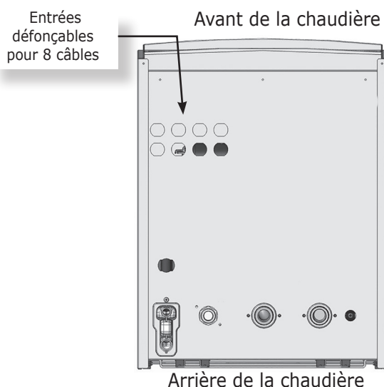
FIGURE 8-1 Entrées défonçables au bas de la chaudière
