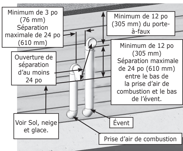
FIGURE 6-16 Événement latéral double (plusieurs appareils)
