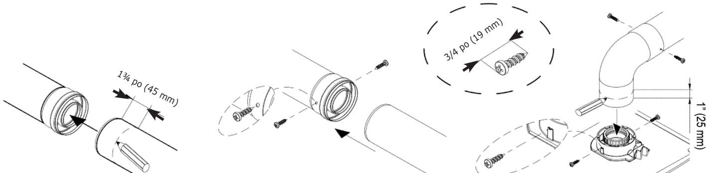
FIGURE 5-4 – Événement coaxial pour installation sur le toit PEUT ÊTRE UTILISÉ SUR TOUTES LES TAILLES
