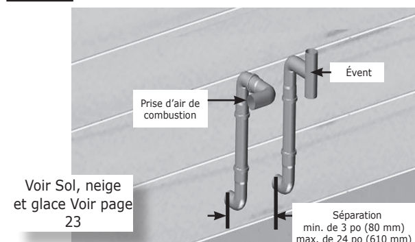
FIGURE 5-32 – (2 po/ 60 mm SEULEMENT) Évent mural latéral pour tuyau double PEUT ÊTRE UTILISÉ SUR TOUTES LES TAILLES
