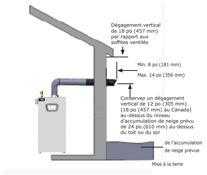
FIGURE 5-7 – Échappement horizontal coaxial - Plusieurs appareils PEUT ÊTRE UTILISÉE SUR TOUTES LES TAILLES
