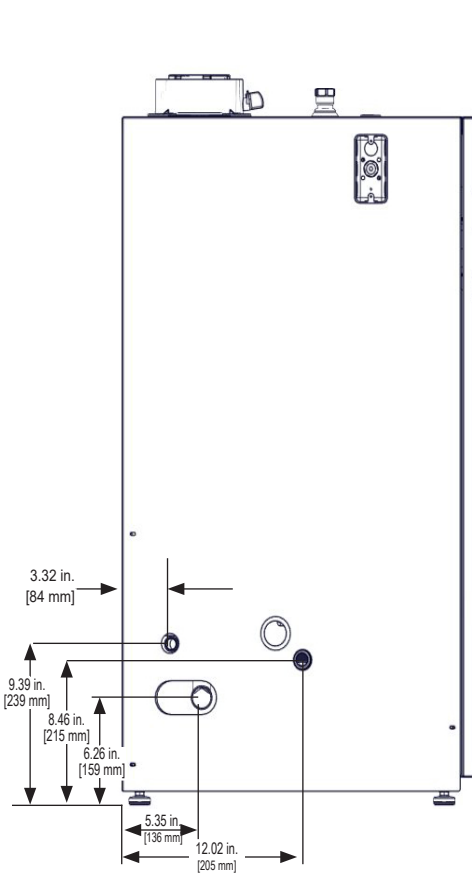
Vue de gauche 165 & 205 Models
