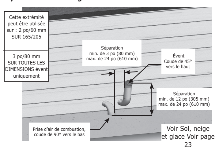
FIGURE 5-27 – (3 po/ 80 mm SEULEMENT) Évent latéral de tuyau double avec angle de 45°
