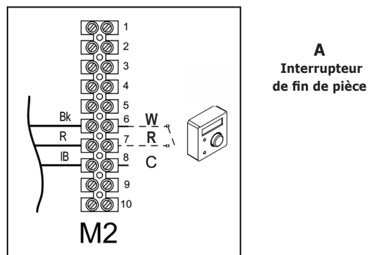
FIGURE 8-4 Raccordements des interrupteurs
