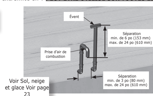
FIGURE 5-31 – (2 po/ 60 mm SEULEMENT) Évent mural latéral pour tuyau double PEUT ÊTRE UTILISÉ SUR TOUTES LES TAILLES
