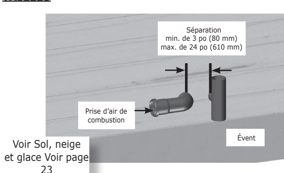
FIGURE 5-32 – (2 po/ 60 mm SEULEMENT) Évent mural latéral pour tuyau double PEUT ÊTRE UTILISÉ SUR TOUTES LES TAILLES
