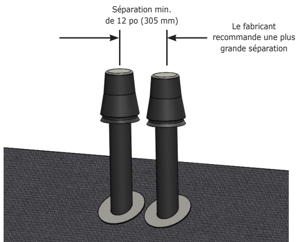
FIGURE 5-5 – Échappement vertical coaxial - Plusieurs appareils PEUT ÊTRE UTILISÉE SUR TOUTES LES TAILLES
