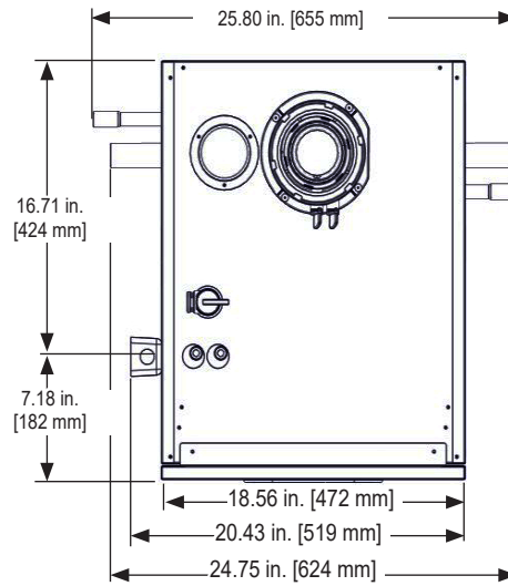
Vue de face 165 & 205 Models
