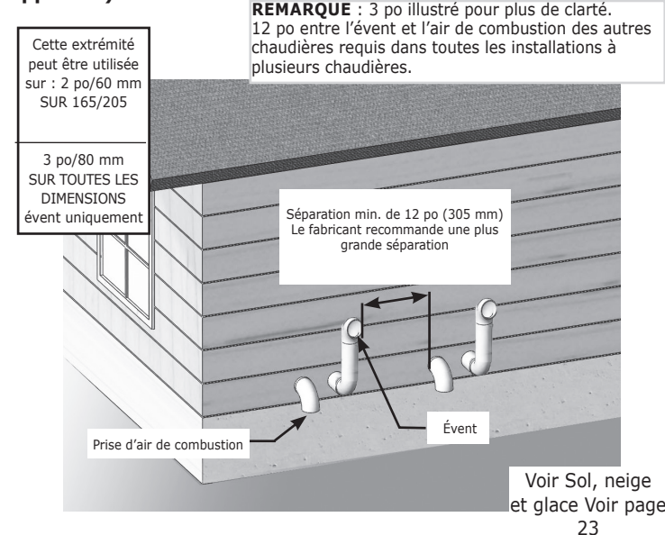
FIGURE 5-27 – (3 po/ 80 mm SEULEMENT) Évent latéral de tuyau double avec angle de 45°
