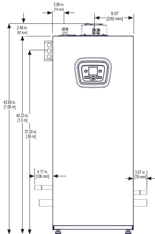
Vue de face 165 & 205 Models
