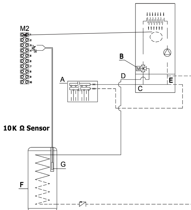
FIGURE 8-7 Réservoir indirect Kt
