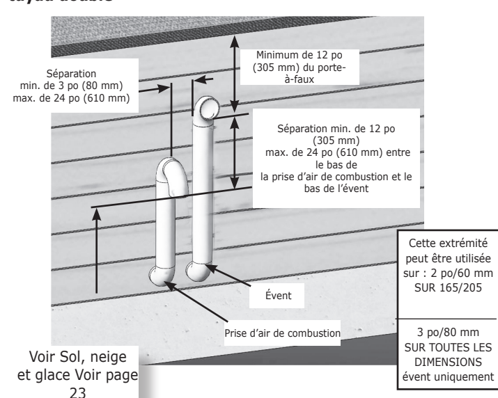
FIGURE 5-28 – (3 po/ 80 mm SEULEMENT) Évent latéral de tuyau double
