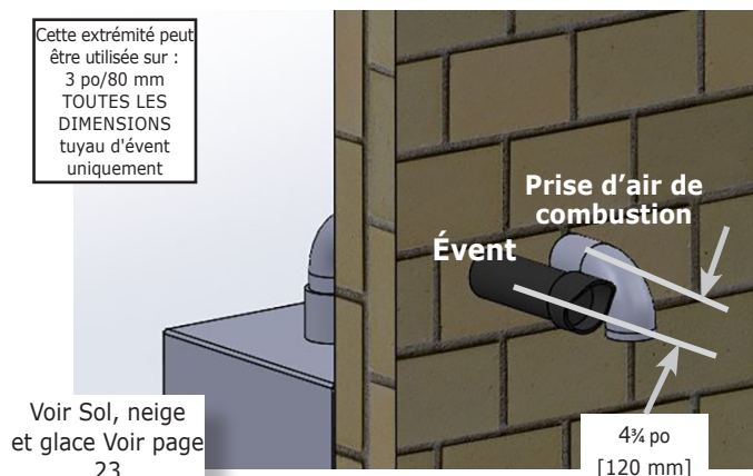
FIGURE 5-24 – (3 po/ 80 mm SEULEMENT) Distance minimale d'un centre à l'autre entre l'adaptateur d'évacuation à paroi simple et la prise d'air
