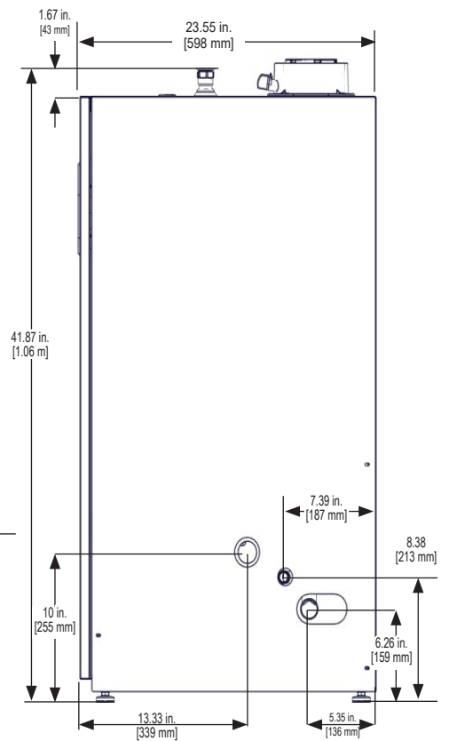
Vue de droite 165 & 205
