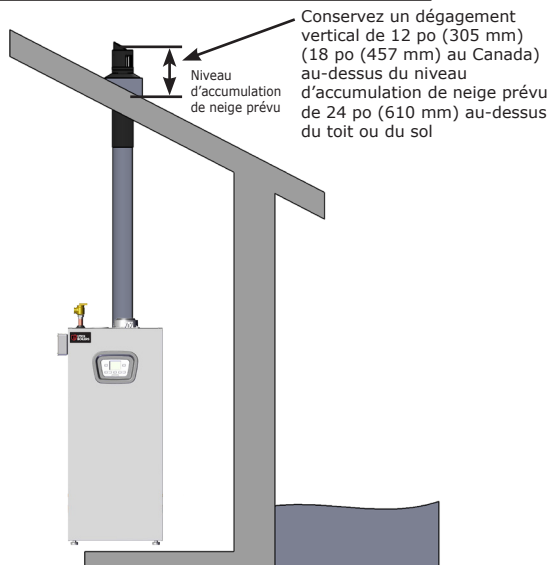
FIGURE 5-4 – Événement coaxial pour installation sur le toit PEUT ÊTRE UTILISÉ SUR TOUTES LES TAILLES
