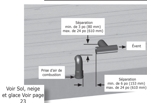
FIGURE 5-30 – (2 po/ 60 mm SEULEMENT) Tuyau d'évent avec extrémité en T PEUT ÊTRE UTILISÉ SUR TOUTES LES TAILLES
