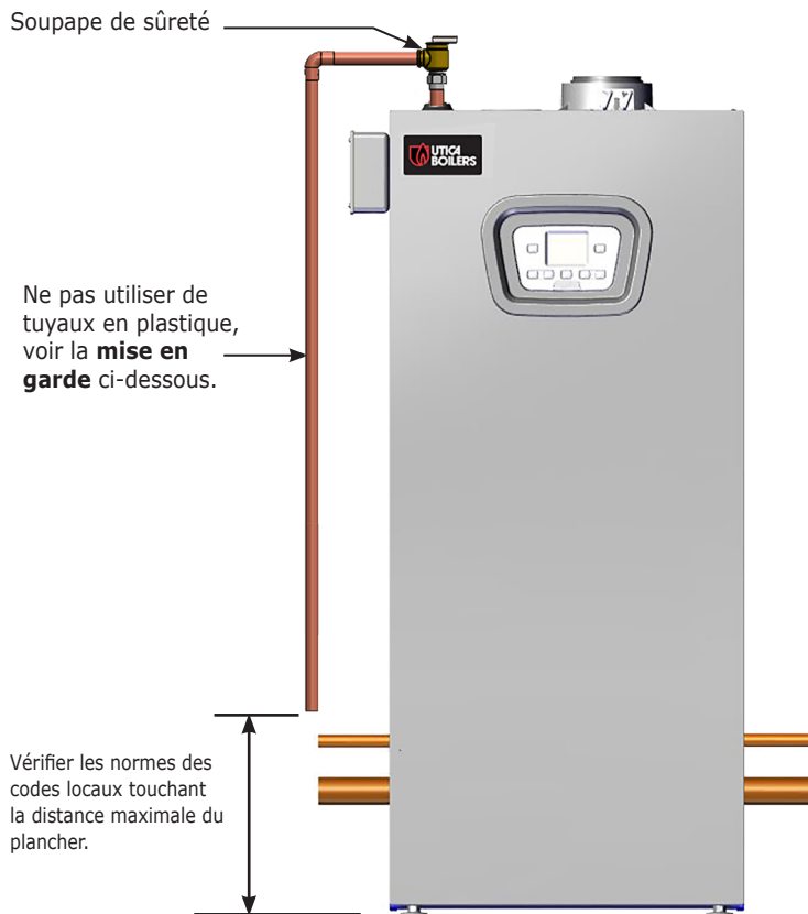
FIGURE 6-1 – Canalisation de sortie de la soupape de sûreté
