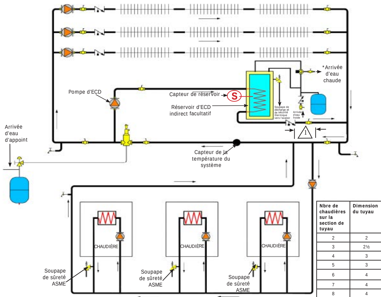
FIGURE 5-7 – Chaudières multiples sans collecteur, avec pompes de zone, primaires et secondaires courantes et indirectes (en option)
