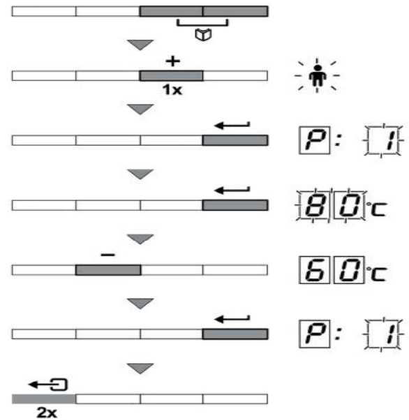
FIGURE 9-10 Paramètres configurables par l'installateur
