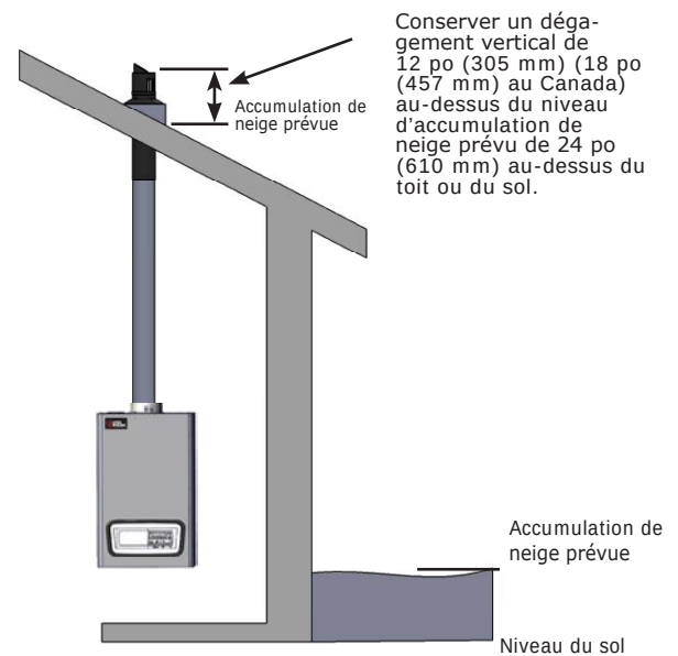
FIGURE 6-3 Événement coaxial pour installation sur le toit
