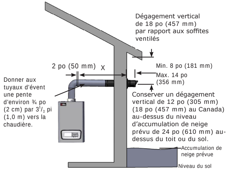
FIGURE 6-2 Événement coaxial pour mur latéral
