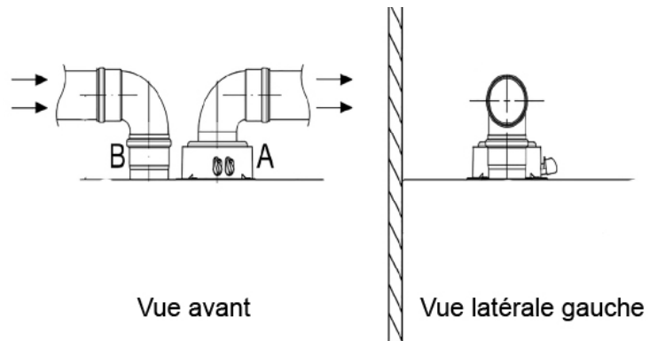
FIGURE 6-6 Options d'installation d'extrémités d'évent horizontales séparées
