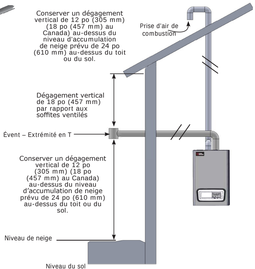
Figure 6-12 Évacuation murale, prise d'air nécessaire à la combustion sur le toit
