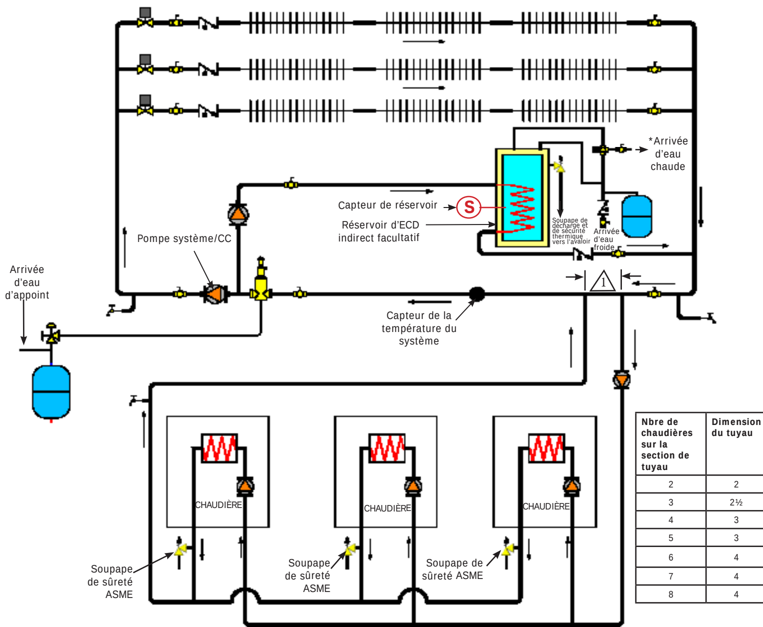
FIGURE 5-6 – Chaudières multiples sans collecteur, avec vannes de zone, primaires et secondaires courantes et indirectes (en option)
