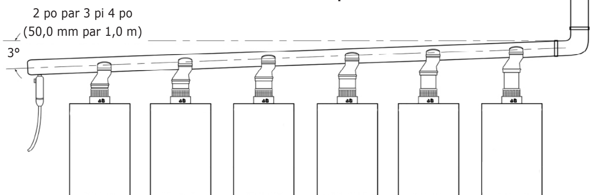
FIGURE 6-26 – Utilisation de ventilation de chaudières multiples
