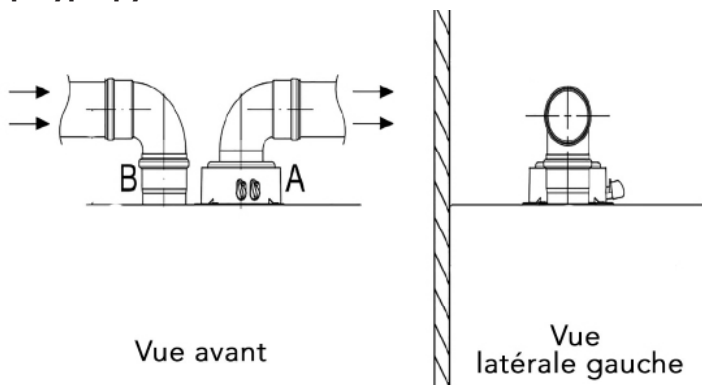
FIGURE 6-3 – Système de tuyau double en polypropylène
