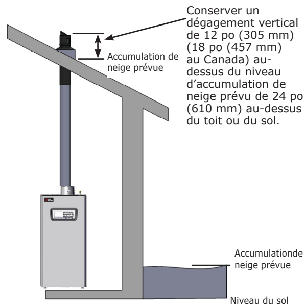
FIGURE 6-2 – Événement coaxial pour installation sur le toit
