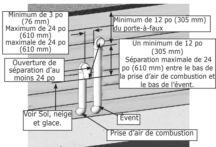
FIGURE 6-8 Évent latéral double (plusieurs appareils)
