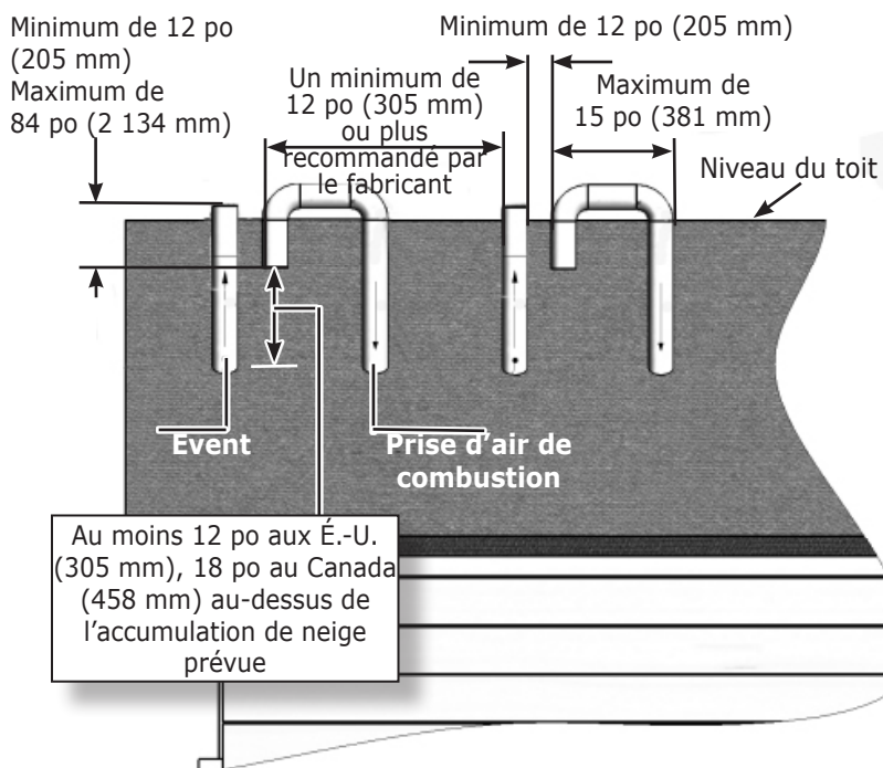
FIGURE 6-7 Évent latéral double
