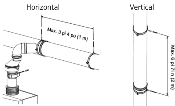
FIGURE 6-24 Distance maximale entre les supports
