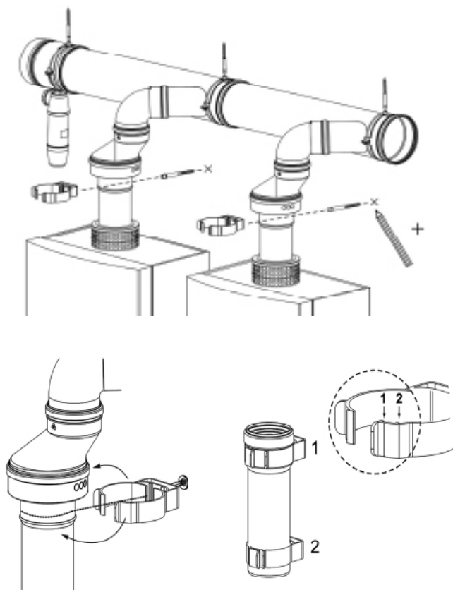
FIGURE 6-23 Fixer la bride autour de l'adaptateur d'évacuation
