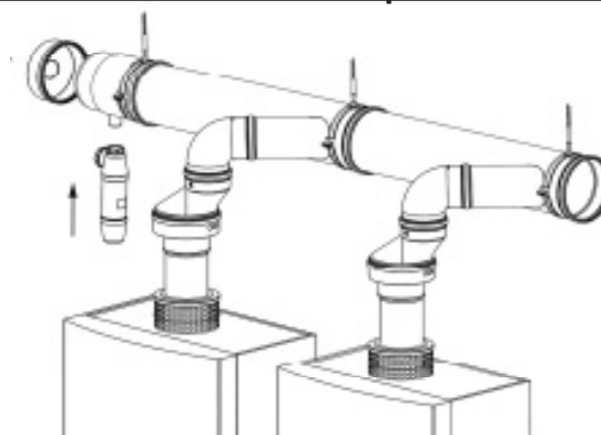
FIGURE 6-22 Installation adéquate des canalisations
