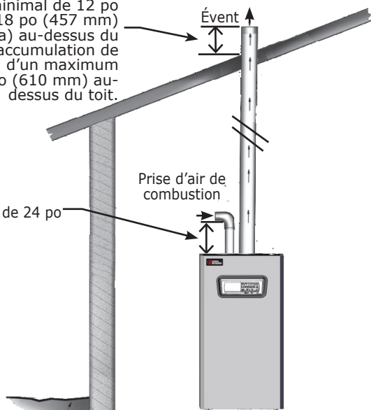
FIGURE 6-12 Évacuation sur le toit, prise d'air nécessaire à la combustion
