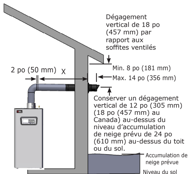
FIGURE 6-1 – Événement coaxial pour mur latéral
