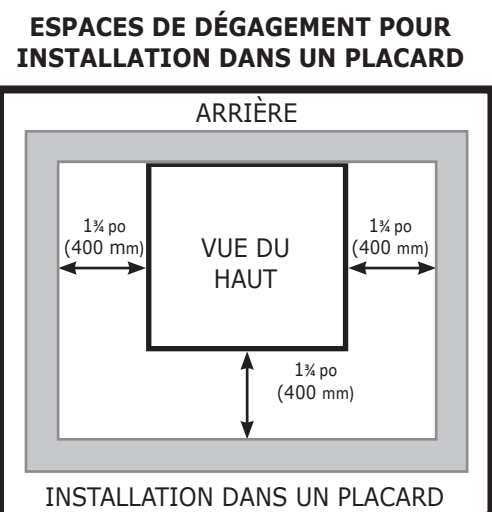
FIGURE 4-2c Dégagement pour le combustible, installation dans un placard
