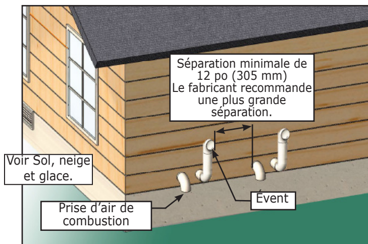
FIGURE 6-8 Évent latéral double (plusieurs appareils)
