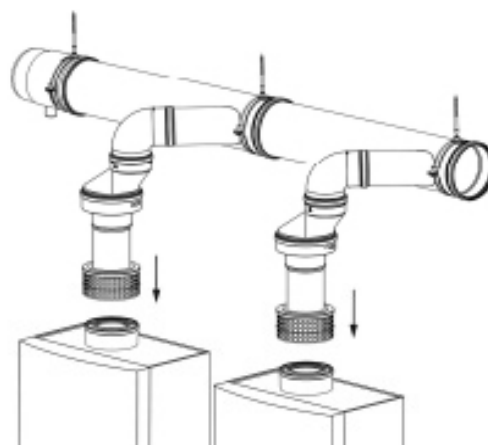
FIGURE 6-22 Installation adéquate des canalisations
