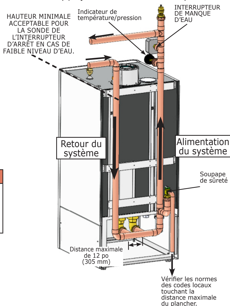
FIGURE 5-3 Indicateur de température/pression et soupape de sûreté
