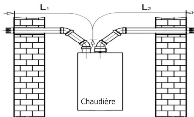
FIGURE 6-4 Options d'installation d'extrémités d'évent horizontales séparées
