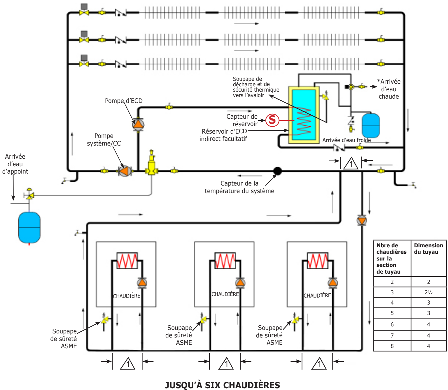
FIGURE 5-6 – Chaudières multiples avec vannes de zone, primaires et secondaires courantes et indirectes (en option)
