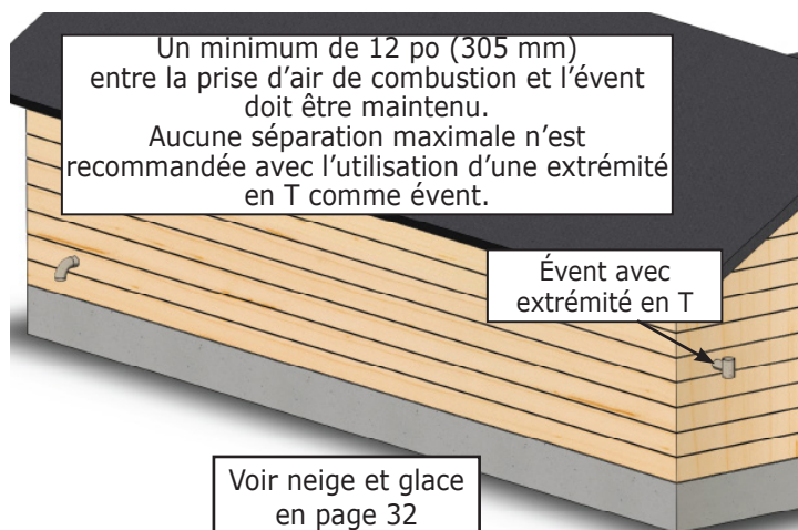
FIGURE 6-9 Extrémité d'évent pour mur latéral avec extrémité en T
