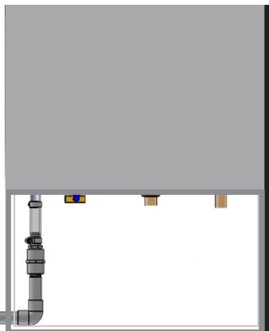
FIGURE 6-29 Tuyau d'écoulement de la condensation
