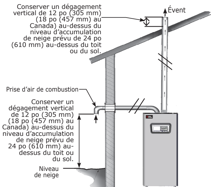
Figure 6-10 Évacuation sur le toit, prise d'air nécessaire à la combustion sur le mur latéral
