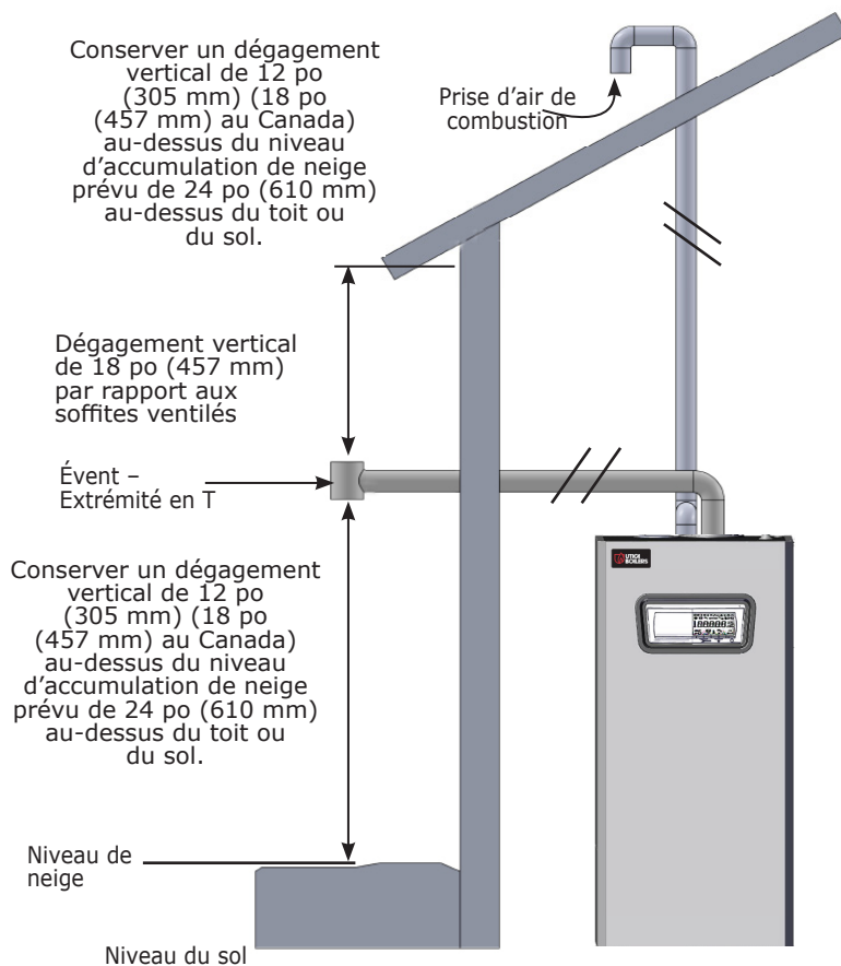
Figure 6-11 Évacuation murale, prise d'air nécessaire à la combustion sur le toit
