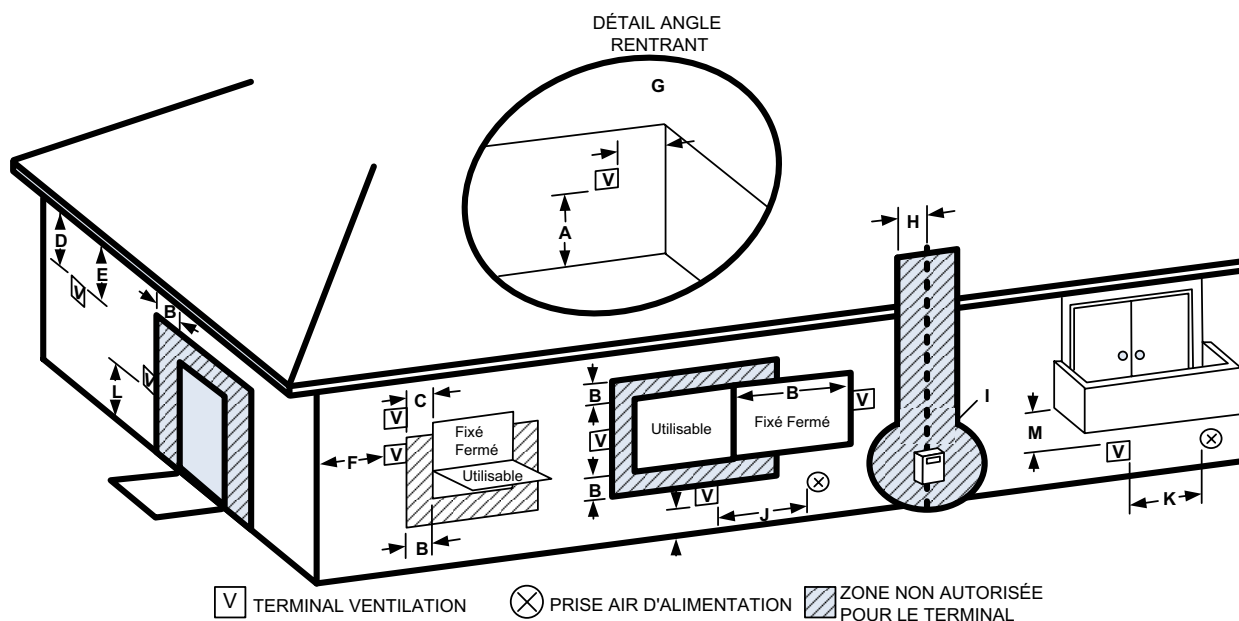
Dégagements minimaux du terminal de ventilation
