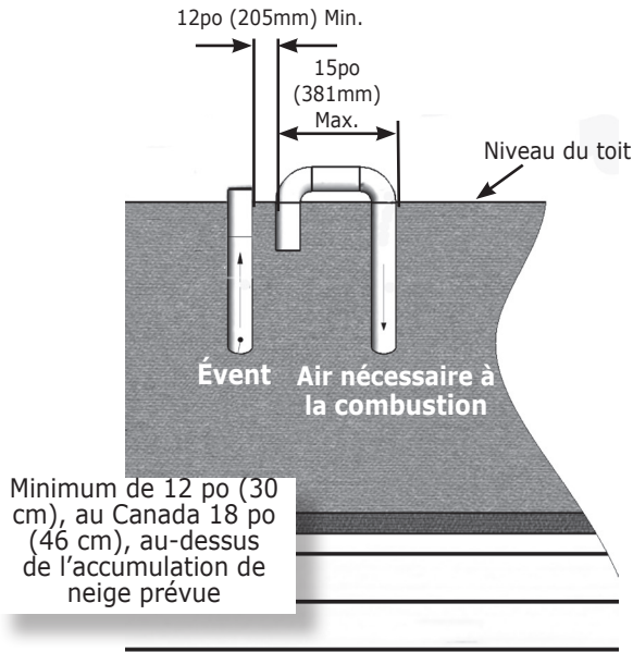
Fig. 7 - Deux tuyaux évent de toit
