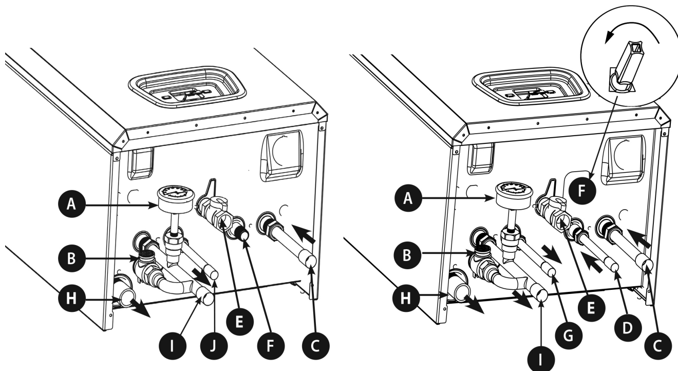
MAH-125
