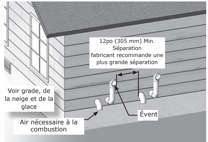
Fig. 9 - Évent de paroi latérale deux tuyaux (plusieurs appliques)
