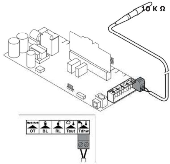
FIGURE 8-12 Thermostat indirect 10 k \Omega pour chauffe-eau
