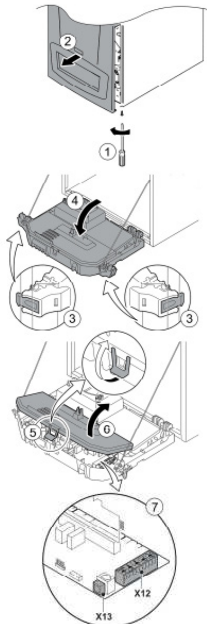
FIGURE 8-2 Retrait du panneau avant
