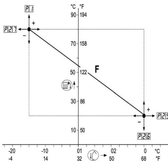
FIGURE 8-11 Tableau du capteur de température extérieure 1k \Omega
