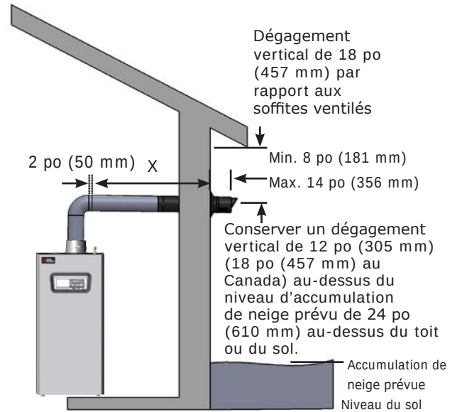
FIGURE 6-2 – Événement coaxial pour mur latéral
