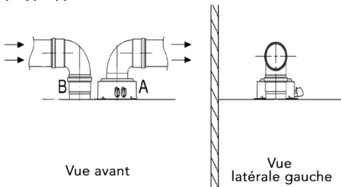
FIGURE 6-5 Adaptateur de système à deux tubes en polypropylène
