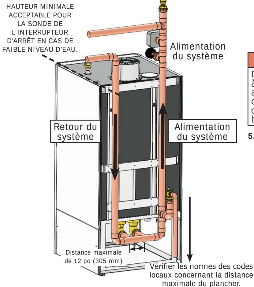
FIGURE 5-2 Canalisations du système : emplacement de la sonde de l'interrupteur en cas de faible niveau d'eau
