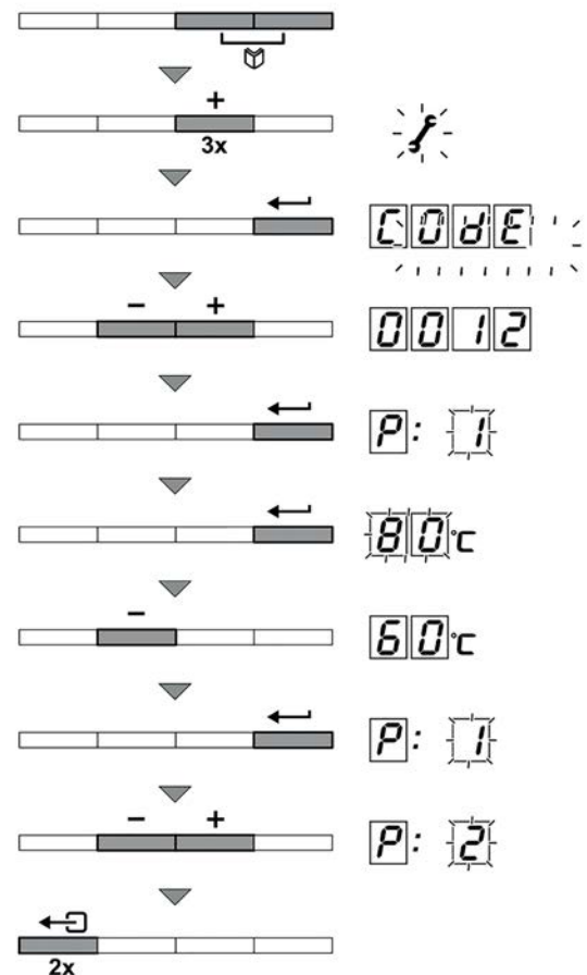
FIGURE 9-8 Paramètres configurables par l'installateur
