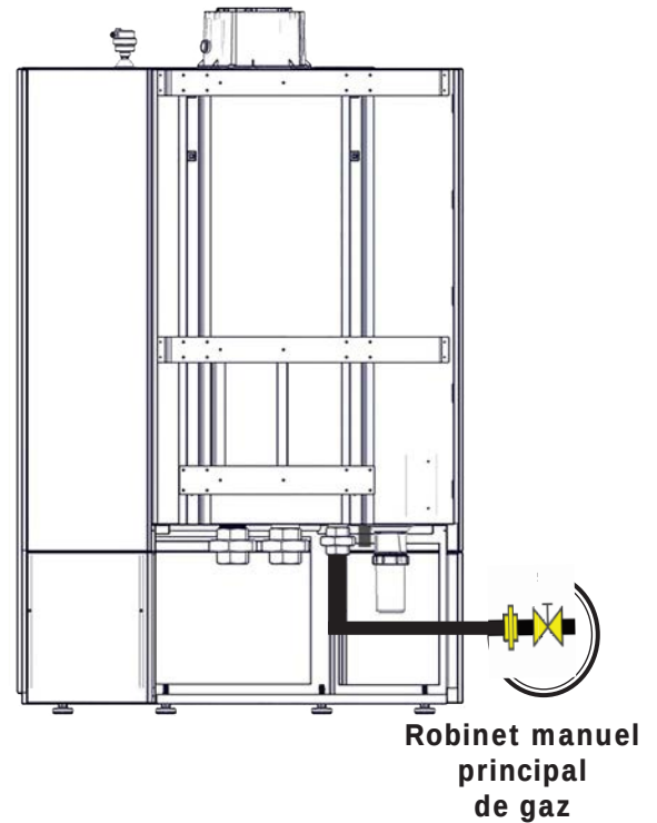
FIGURE 7-3 Robinet manuel principal d'approvisionnement en gaz à l'extérieur de la paroi de la chaudière - (vue de l'arrière de la chaudière)
