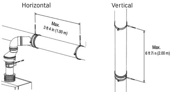
FIGURE 6-25 Distance maximale entre les supports
