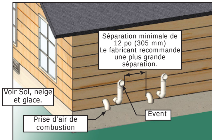
FIGURE 6-9 Événement latéral double (plusieurs appareils)
