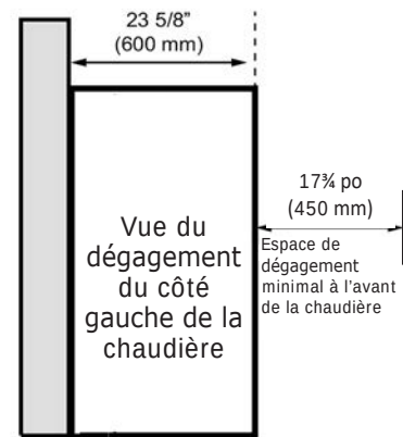
FIGURE 4-2b Dégagement pour l'entretien, vue côté gauche de la chaudière
