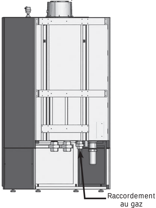
FIGURE 7-1 Raccordement au gaz (vu de l'arrière de la chaudière)
