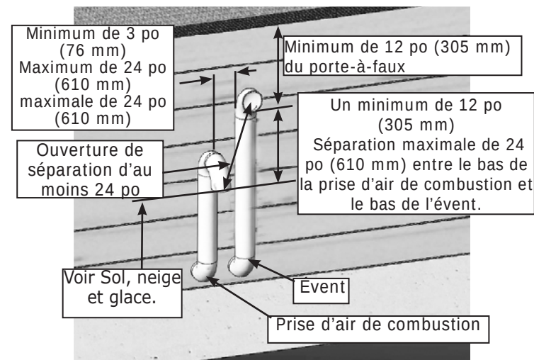
FIGURE 6-9 Événement latéral double (plusieurs appareils)
